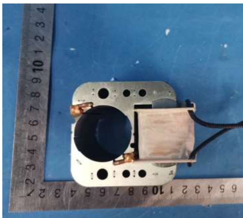
S60H-A13 定子
