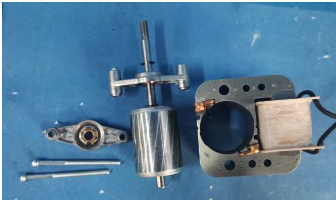
S60H-A13 内部结构
