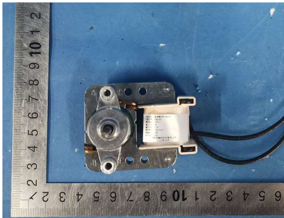
S48H-A02 外观
