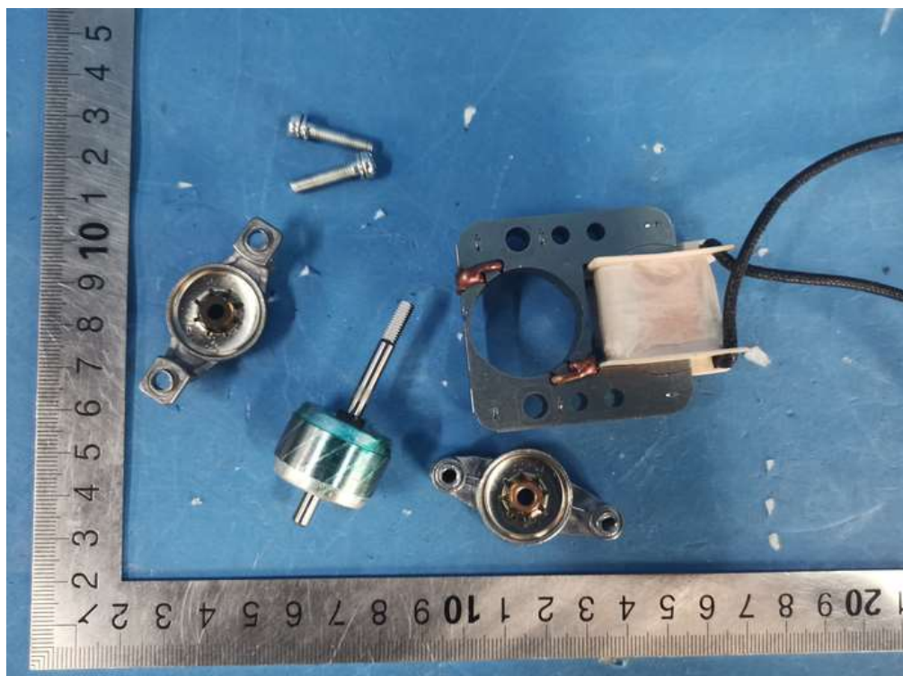
S48H-A02 内部结构
