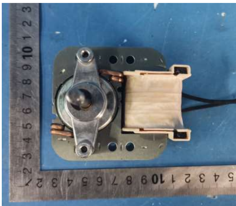
S60H-A13 外观
