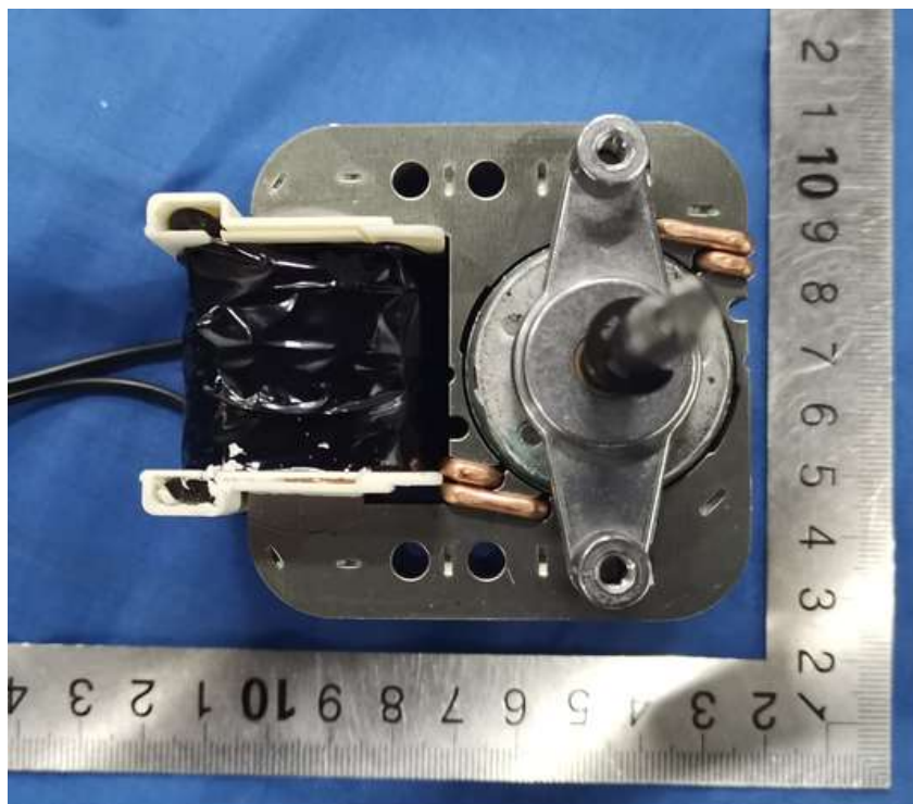
外观
