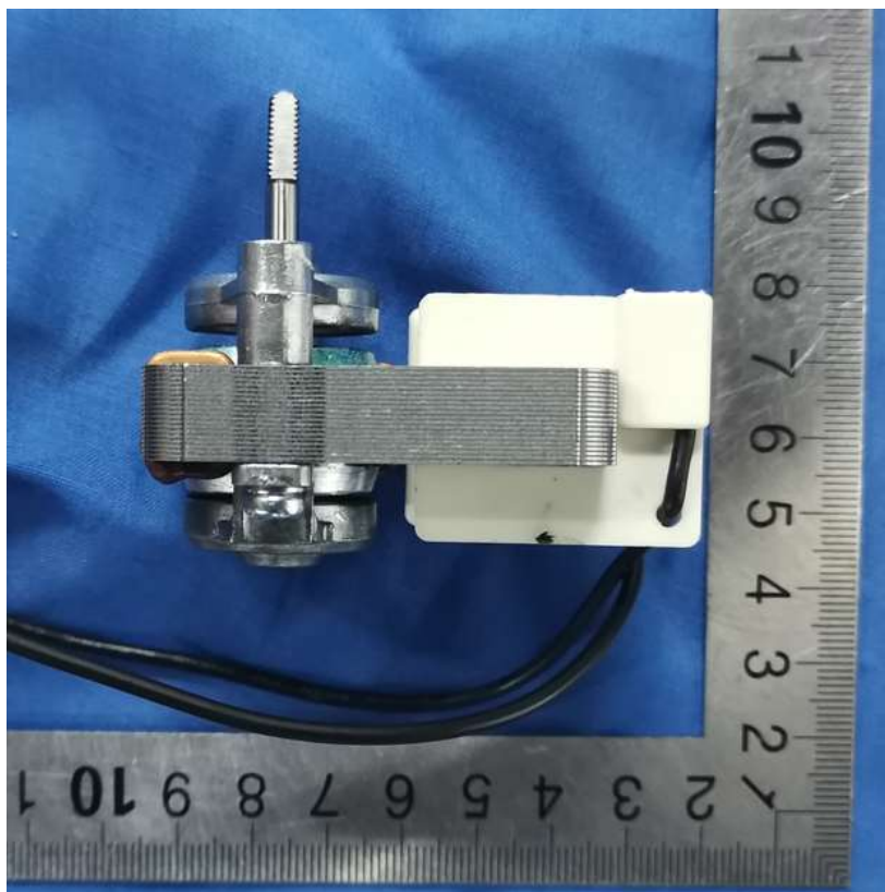
外观
