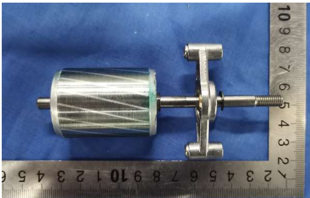
转子
