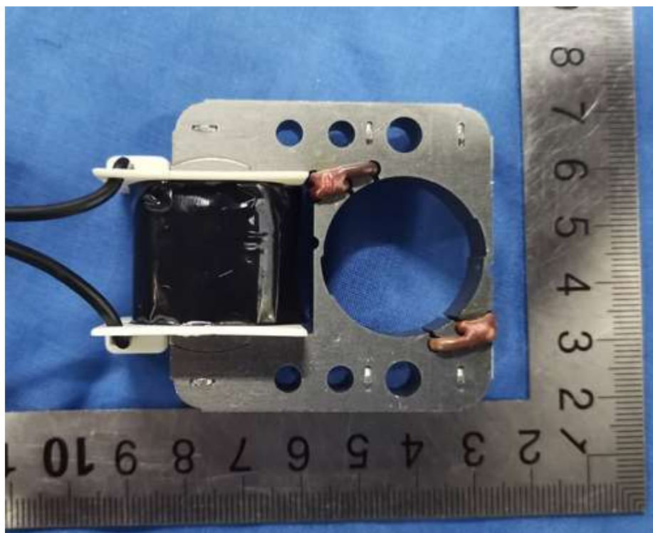
定子
