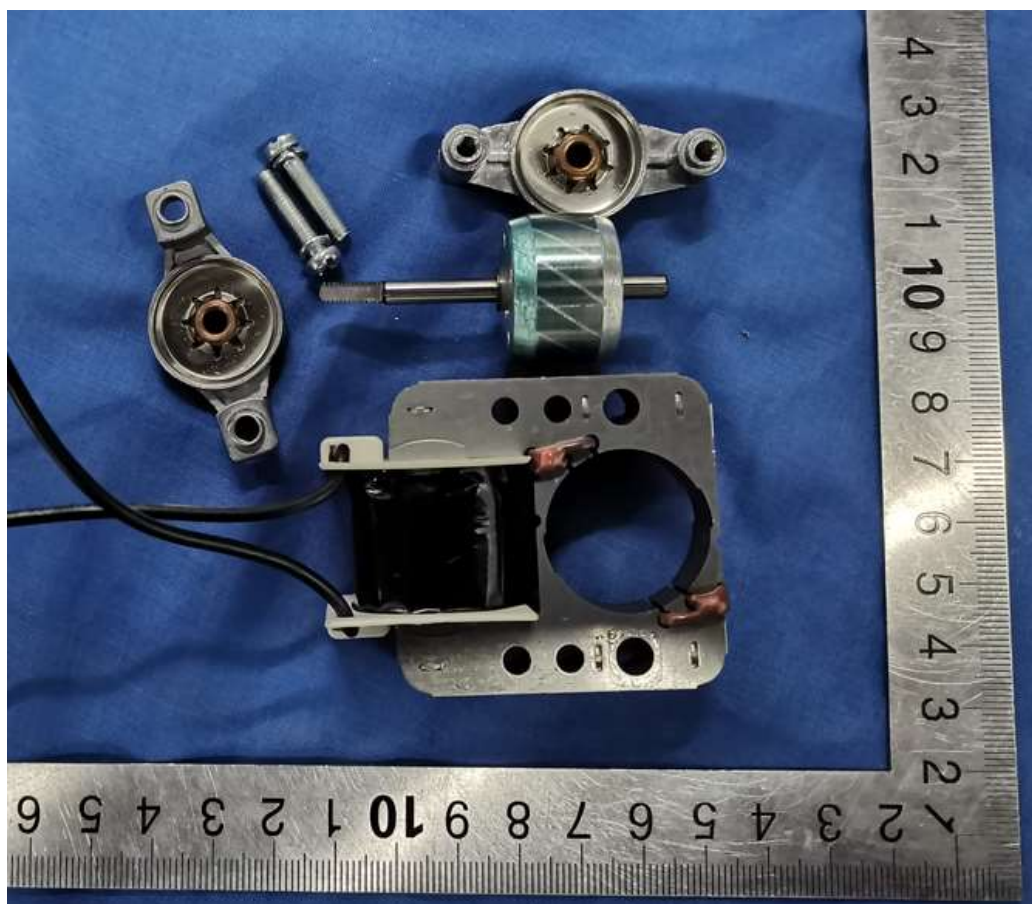
内部结构
