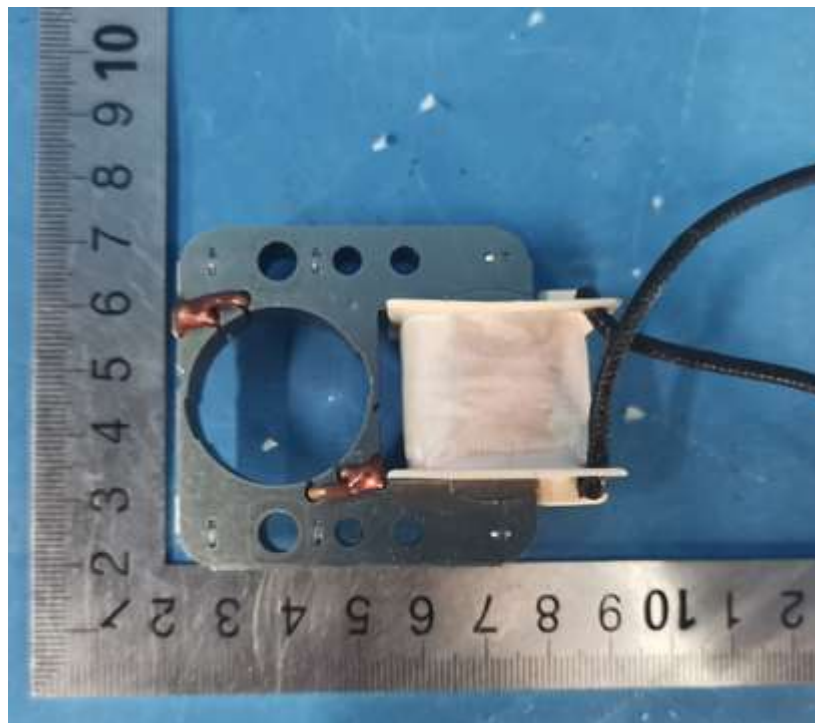
定子
