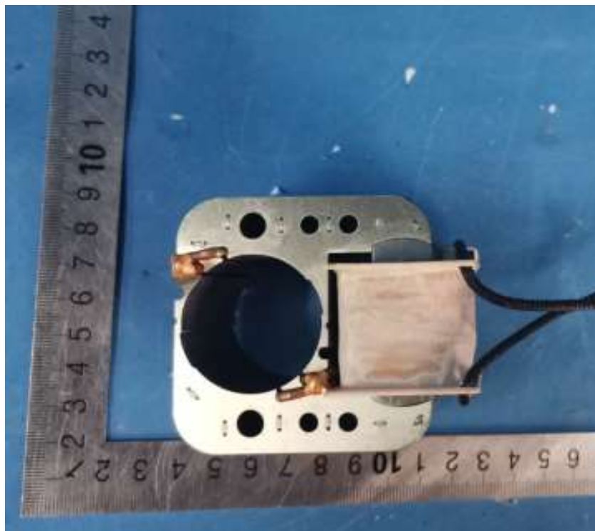
定子
