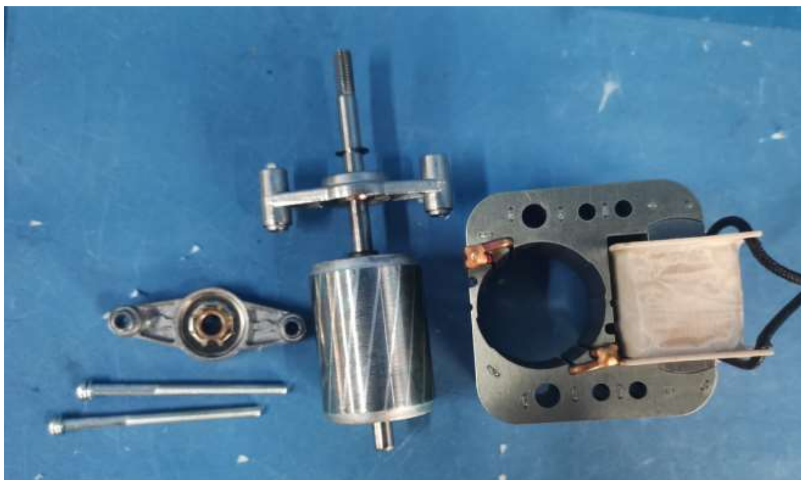
内部结构
