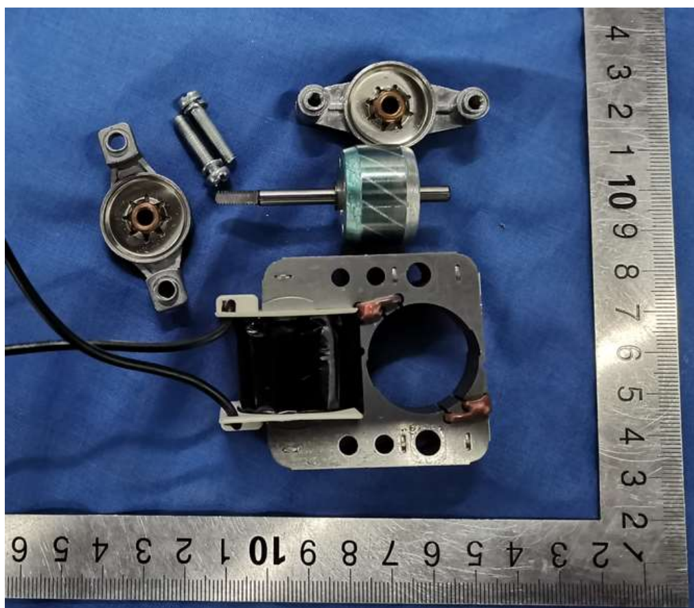
内部结构
