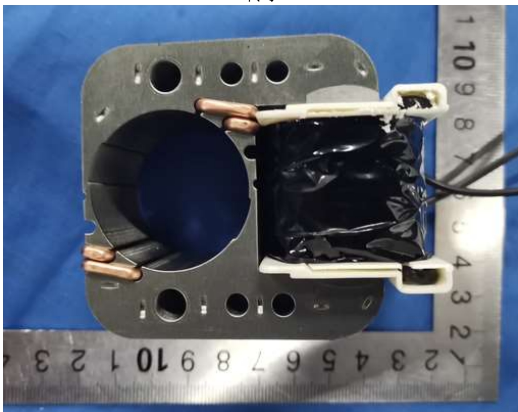
定子
