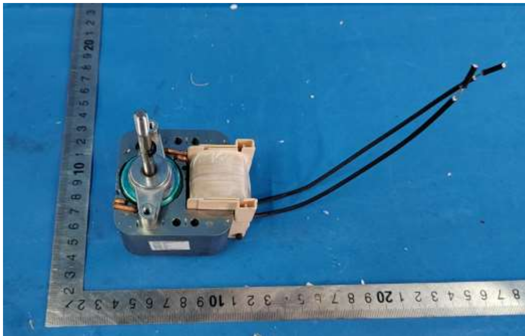
S60H-B13-LX 外观
