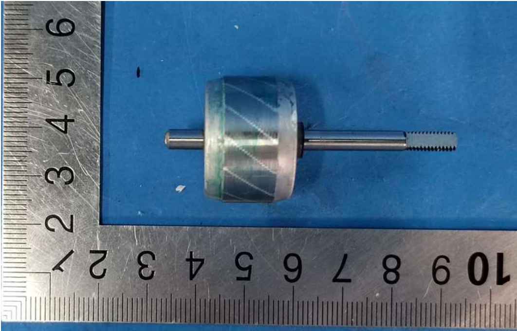
S48H-B01-LX 转子
