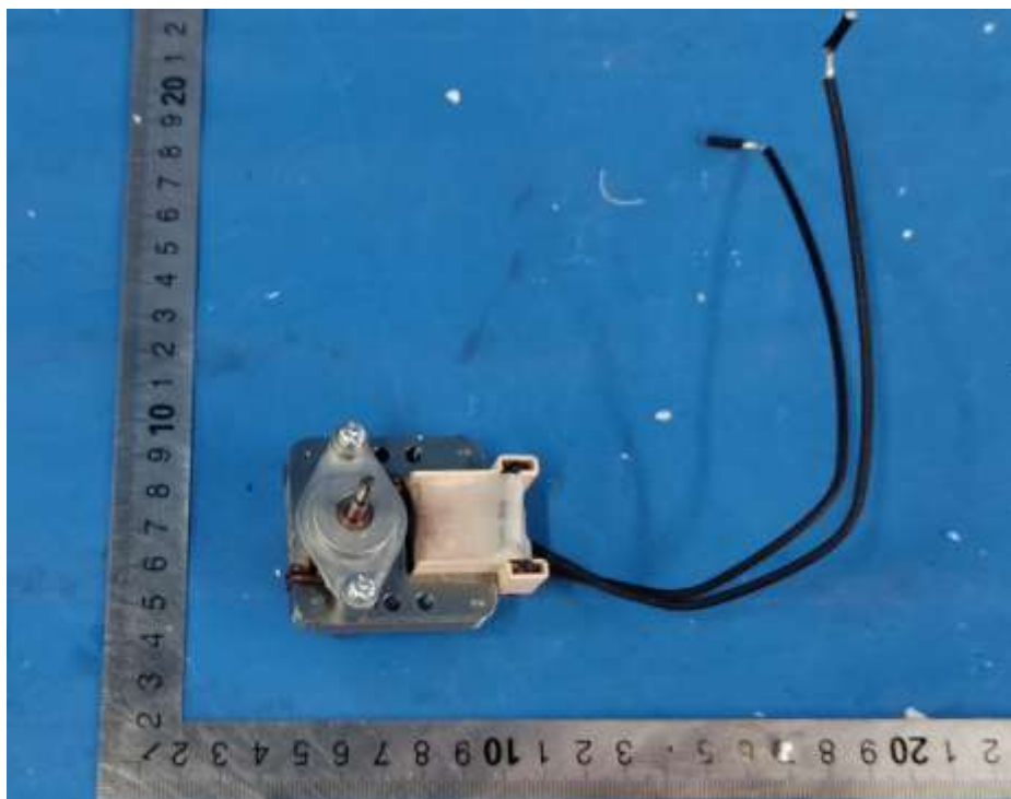
S48H-B01-LX 外观
