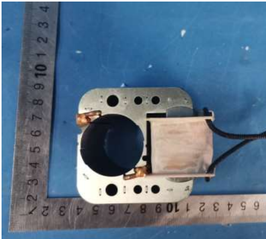
S60H-A13-LX 定子
