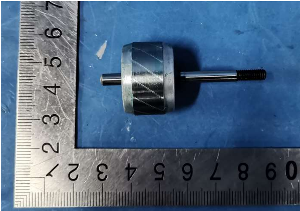
S48H-A01-LX 转子
