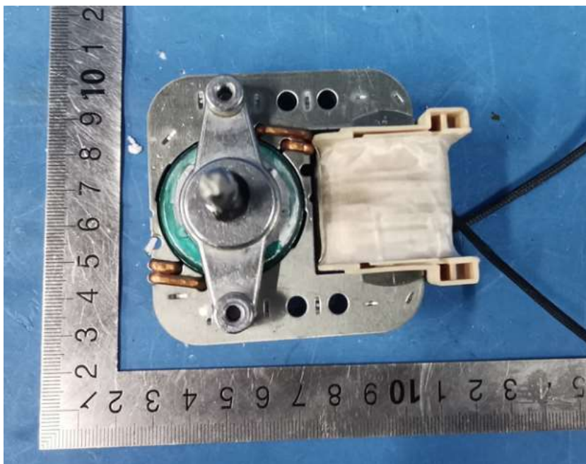
S60H-A13-LX 外观
